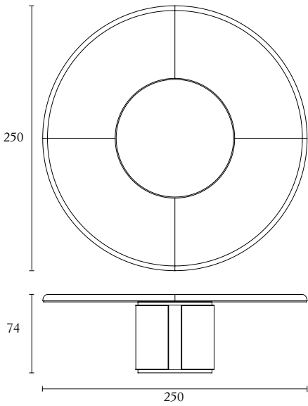
Cod. HELYTA250 cm Ø 250 x h 74 - inch 98.4 x 29.1
